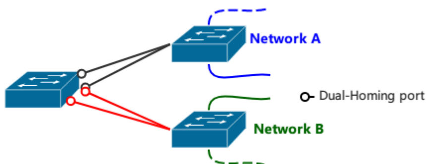
Рисунок 14-20: Подключение дуал-хоминг к сегментам А и В
