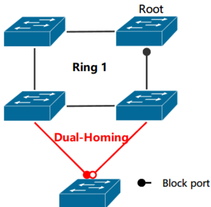
Рисунок 14-6: Схема топологии DG-Ring с двумя ведущими устройствами и резервированием линий связи.
