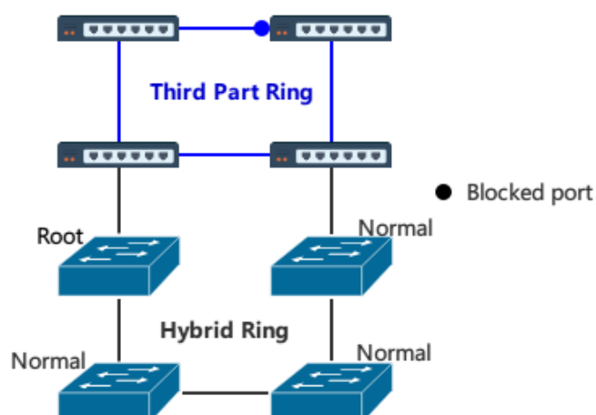
Рисунок 14-21: Комбинированная работа гибридного кольца и кольца стороннего производителя
