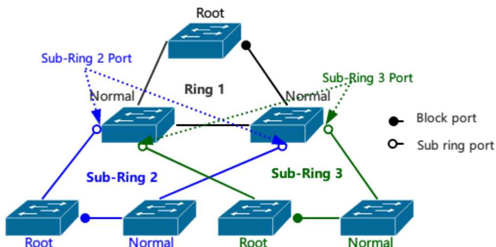
Рисунок 14-16: Схема сети с пересекающимися кольцами DG-Ring (вариант 1)
