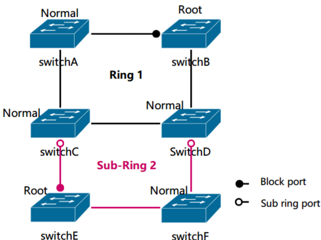
Рисунок 14-1: Схема принципа работы DG-Ring.
