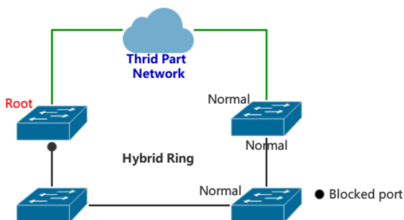
Рисунок 14-7: Схема подключения и настройки Hybrid-Ring.
