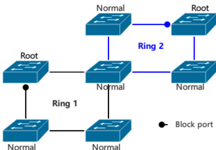
Рисунок 14-15: Схема сети с касательными кольцами DG-Ring
