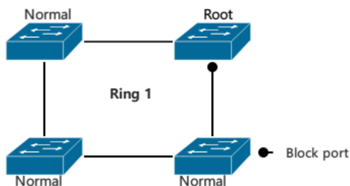
Рисунок 14-14: Схема сети с одиночным кольцом DG-Ring
