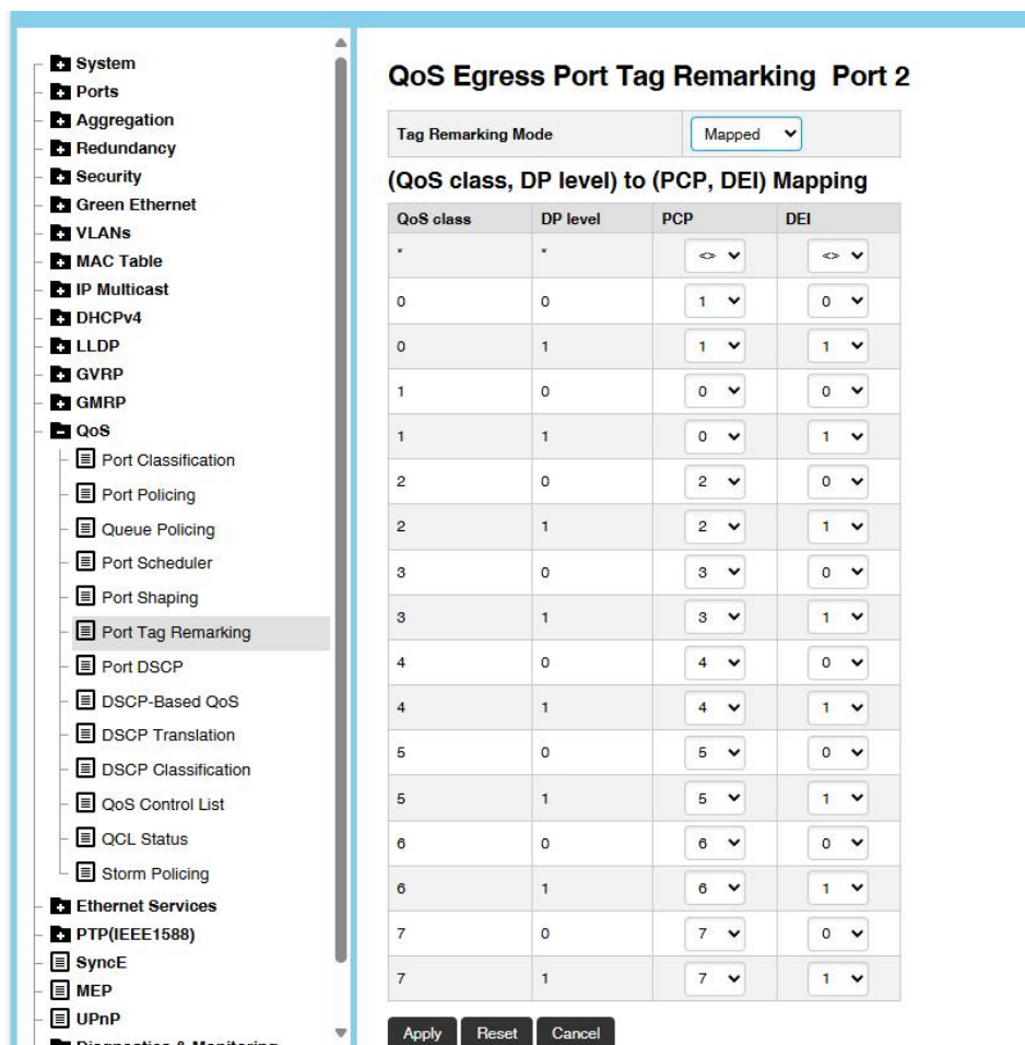
Рисунок 6-3: Маркировка исходящего порта QoS
