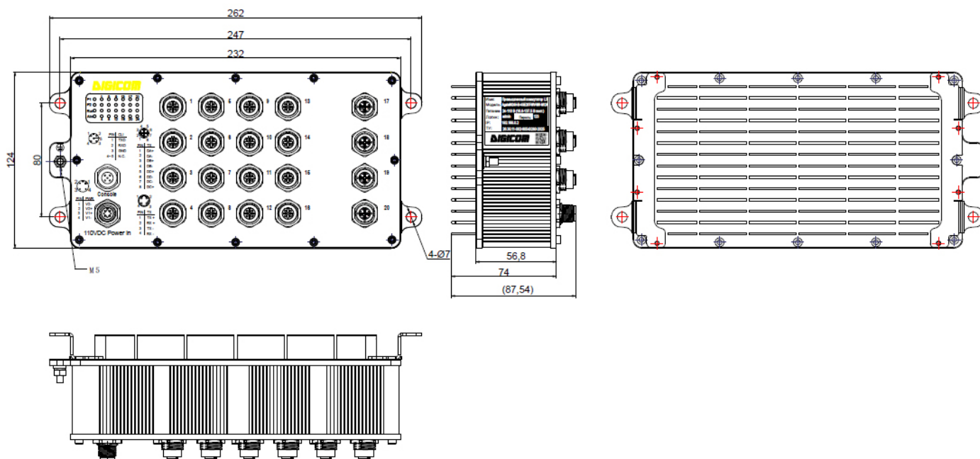
Рисунок 1 – коммутатор Agate8620H
